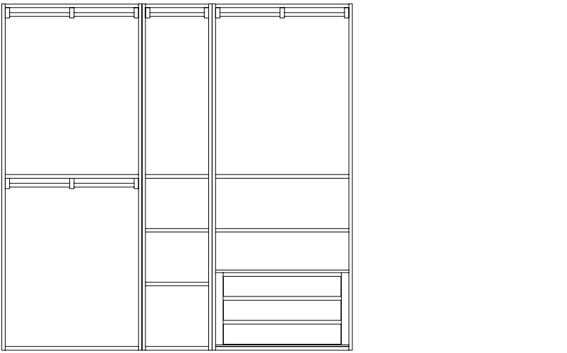
Articolo 4466 Proposta componibile cabina armadio (doppio fianco) predisposta per inserimento ante, esterno in frassino interno in tanganica. Modular walk-in wardrobe proposal (double side) designed for the insertion of doors, exterior in ash, interior in Tanganyika. cm. L. 250 P. 59 H.247
