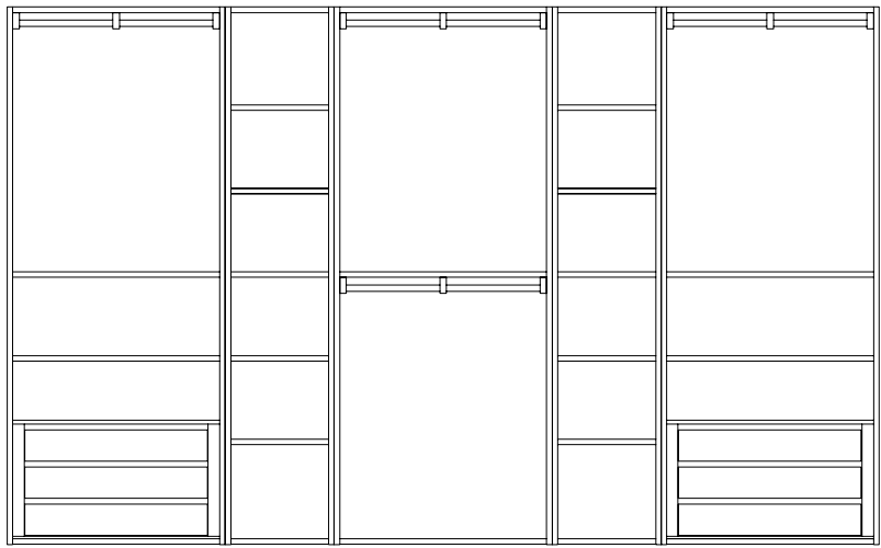
Articolo 4463.B Proposta componibile cabina armadio (doppio fianco) predisposta per inserimento ante, esterno in frassino interno in tanganica. Modular walk-in wardrobe proposal (double side) designed for the insertion of doors, exterior in ash, interior in Tanganyika. cm. L. 400 P. 59 H.247
