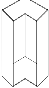
Articolo 4472.F Articolo 4472.T struttura angolo 90° 2 ante passo ripiani in h.16,7 cm. cm. 111,8 x 111,8/59 h.247
