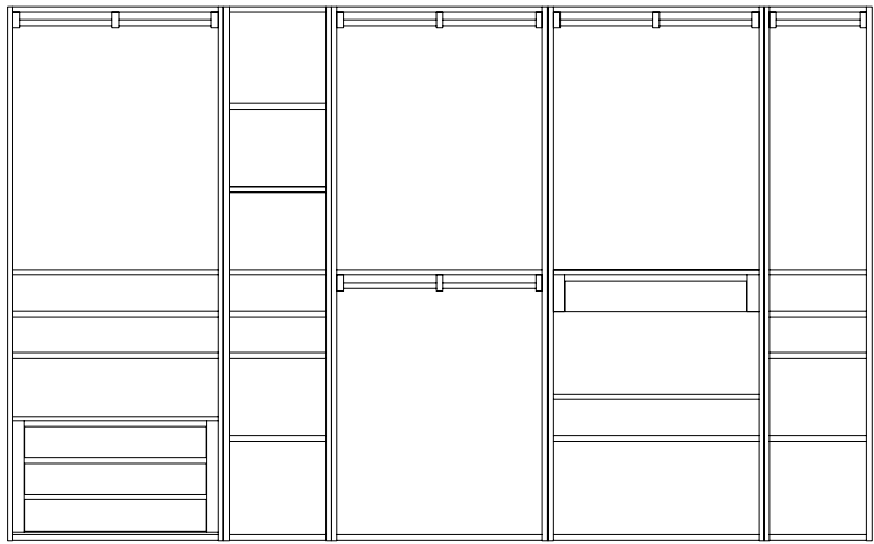
Articolo 4463.A Proposta componibile cabina armadio (doppio fianco) predisposta per inserimento ante, esterno in frassino interno in tanganica. Modular walk-in wardrobe proposal (double side) designed for the insertion of doors, exterior in ash, interior in Tanganyika. cm. L. 400 P. 59 H.247
