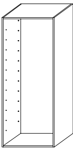
Articolo 4467.F Articolo 4467.T struttura cabina armadio doppia passo ripiani in h.16,7 cm. cm. 100 x 59 h.247
