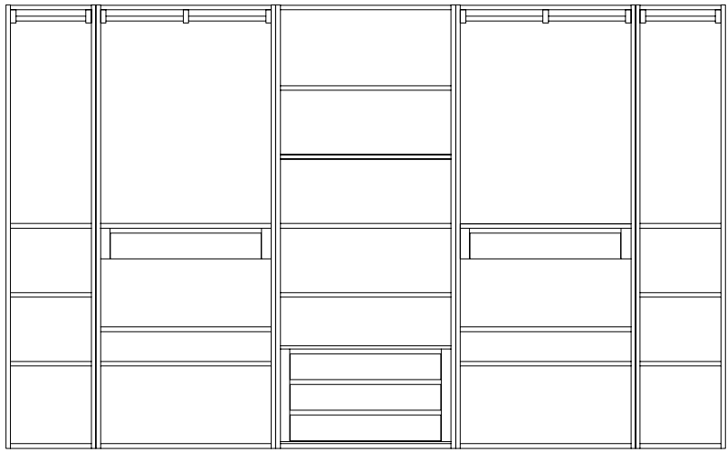
Articolo 4463.C Proposta componibile cabina armadio (doppio fianco) predisposta per inserimento ante, esterno in frassino interno in tanganica. Modular walk-in wardrobe proposal (double side) designed for the insertion of doors, exterior in ash, interior in Tanganyika. cm. L. 400 P. 59 H.247
