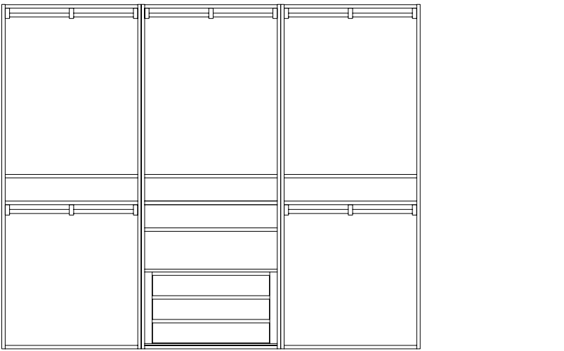
Articolo 4465 Proposta componibile cabina armadio (doppio fianco) predisposta per inserimento ante, esterno in frassino interno in tanganica. Modular walk-in wardrobe proposal (double side) designed for the insertion of doors, exterior in ash, interior in Tanganyika. cm. L. 300 P. 59 H.247
