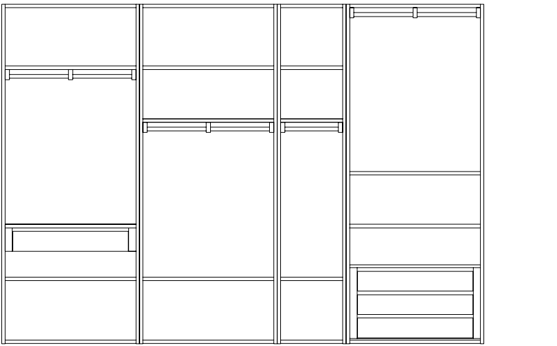
Articolo 4464 Proposta componibile cabina armadio (doppio fianco) predisposta per inserimento ante, esterno in frassino interno in tanganica. Modular walk-in wardrobe proposal (double side) designed for the insertion of doors, exterior in ash, interior in Tanganyika. cm. L. 350 P. 59 H.247
