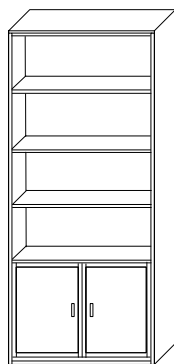
Articolo 2908 Colonna doppia. Column. cm. L. 94,5 P. 35 H. 225
