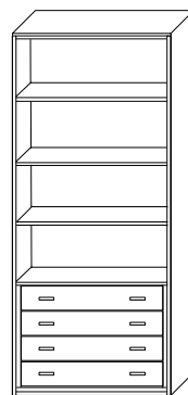
Articolo 2910 Colonna doppia. Column. cm. L. 94,5 P. 35 H. 225
