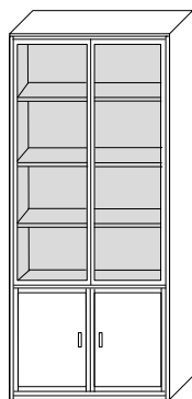
Articolo 2909 Colonna doppia. Column. cm. L. 94,5 P. 35 H. 225
