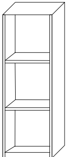
Articolo 3120 Colonna componibile solo scocca. Body only modular column. cm. L. 60 P. 39 H. 182,5
